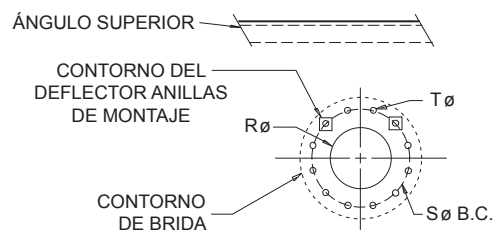
DETALLE CORTE DE TANQUE PARA CÁMARA DE ESPUMA MCS-55
