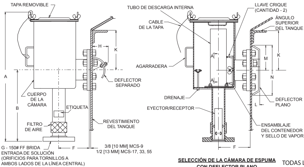
CÁMARA DE ESPUMA CON DEFLECTOR SEPARADO
