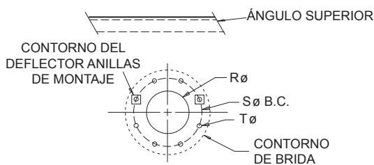
DETALLE CORTE DE TANQUE PARA CÁMARA DE ESPUMA MCS-9, MCS-17 & MCS-33
