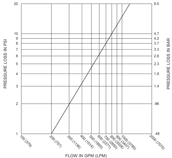
MONITOR MMB-3 X 2-1/2 CUADRO DE PRESIÓN VS. CAUDAL
