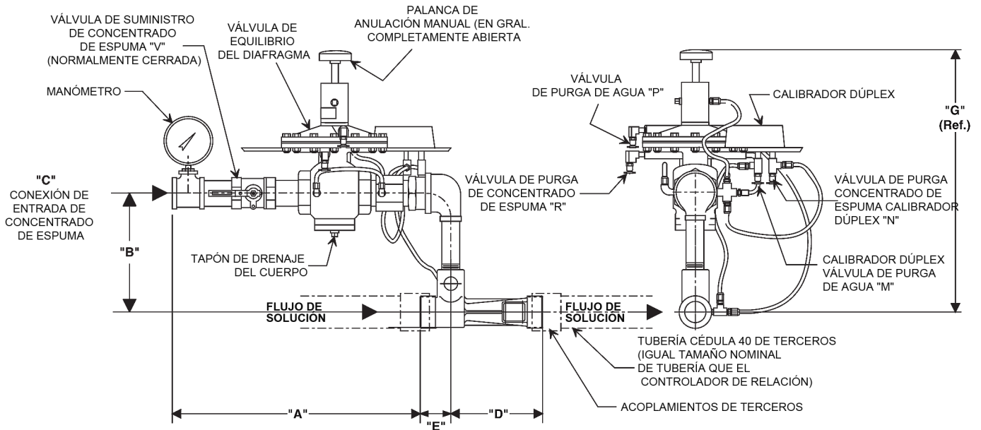
Módulo de proporciónamiento de presión balanceada en línea con anulación manual
